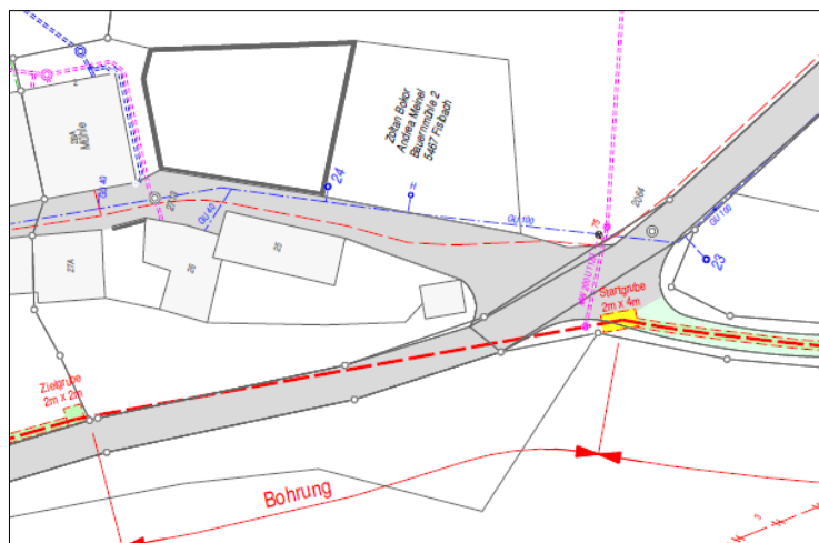
Ausschnitt Projekt Ersatz Freileitung TS Lochmühle – TS Dorf
